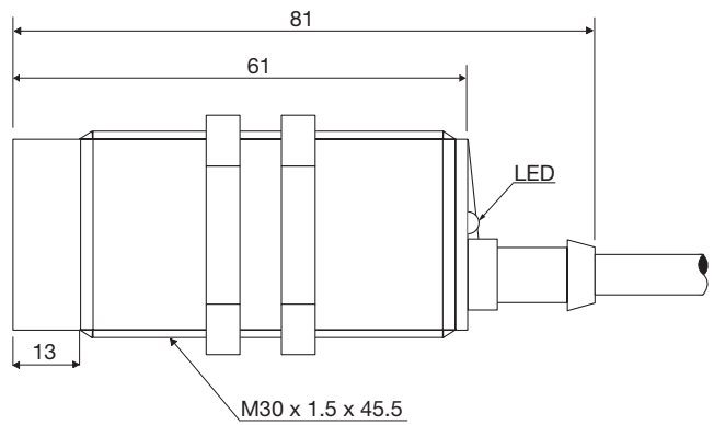
Fig. 7 Kabel CA30CAN...A2IO
