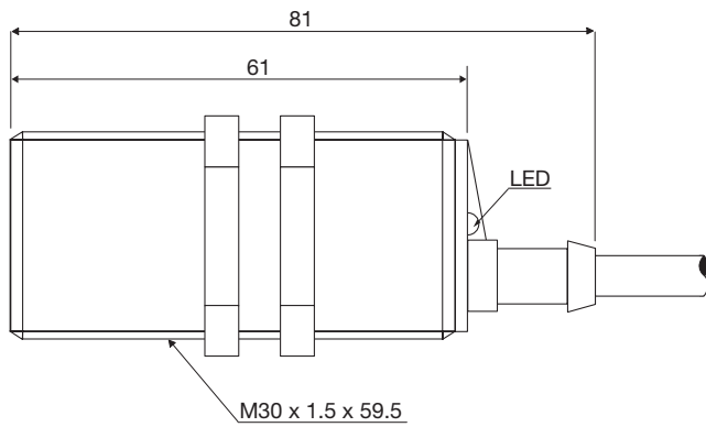
Fig. 6 Kabel CA30CAF...A2IO
