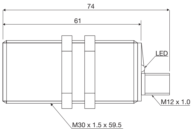
Fig. 8 Stik CA30CAF...M1IO
