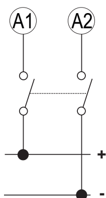
Fig. 1 Strømforsyning
