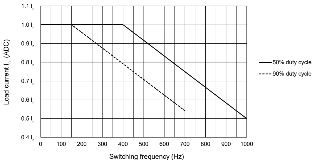
Fig. 5 Strømbegrænsning vs. skiftfrekvens 4
