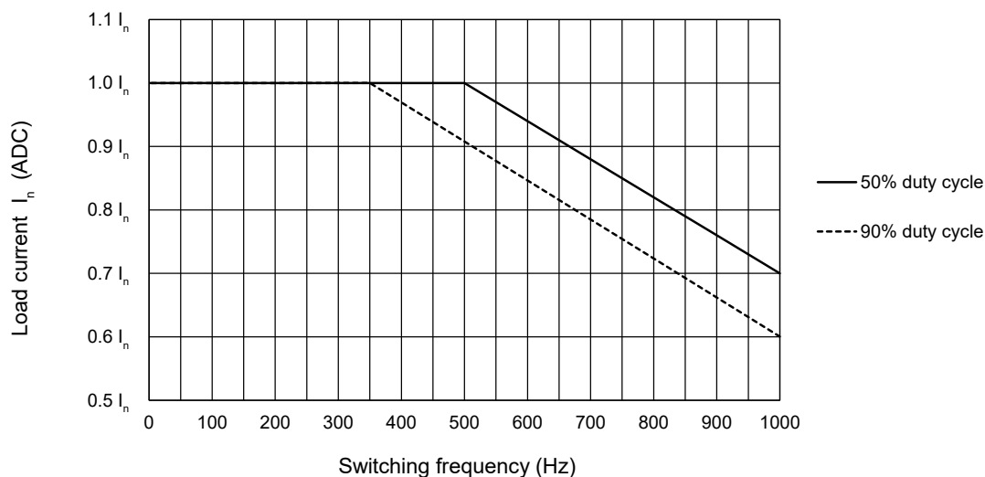
Fig. 4 Strømbegrænsning vs. skiftfrekvens
