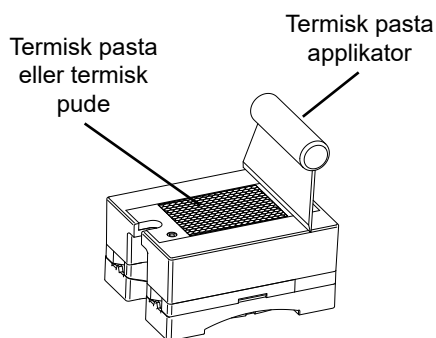
Fig. 12 Et fint lag termisk ledende silicumpasta skal fordeles jævnt på SSR-basen, før montering på en køleplade. Alternativt kan man anvende en termisk plade. Materialet i den termiske interface påvirker den termiske ydelse. Sørg for, at kølepladen har den rette størrelse.
