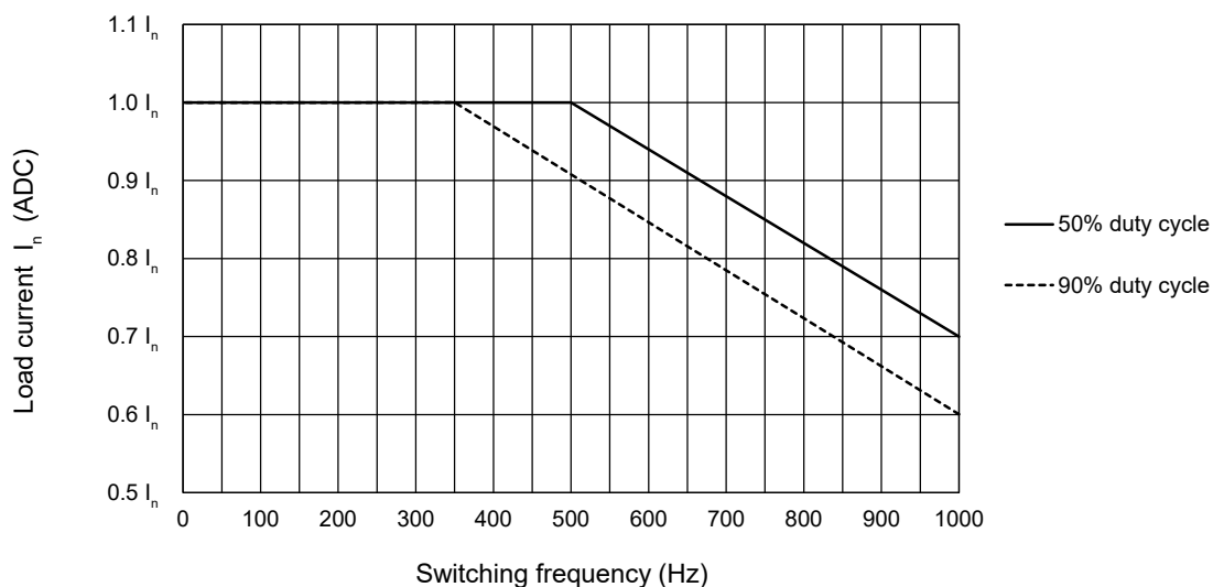
Fig. 4 Strom-Derating und Schaltfrequenz
