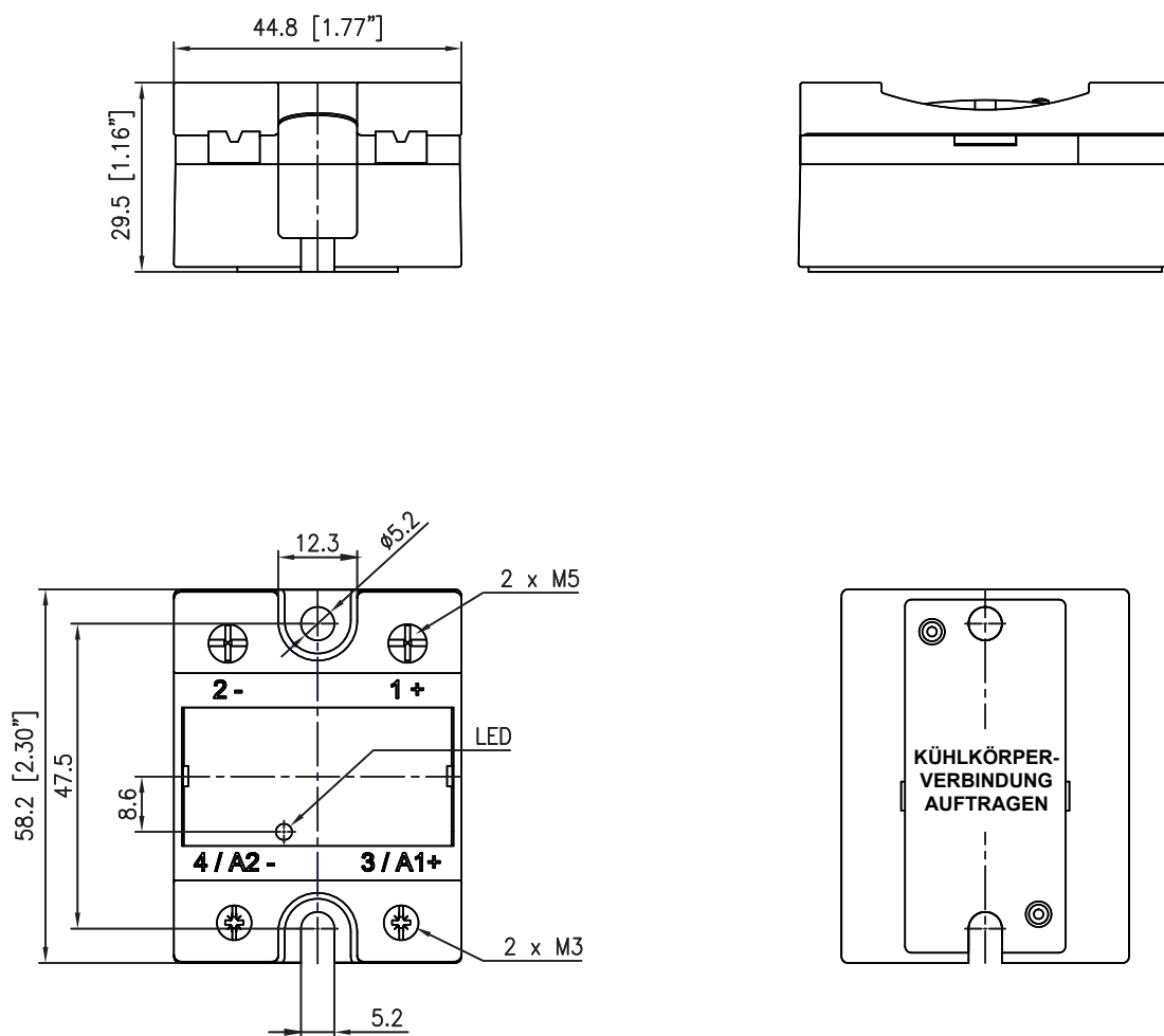
Fig. 1 RM1D Abmessungen
