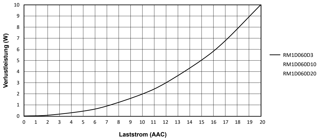
Fig. 7 Verlustleistungskurve
