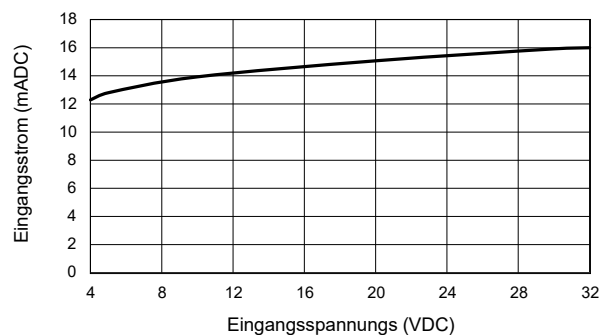
Fig. 3 Eingangsspannungs-Eingangsstrom-Kennlinie
