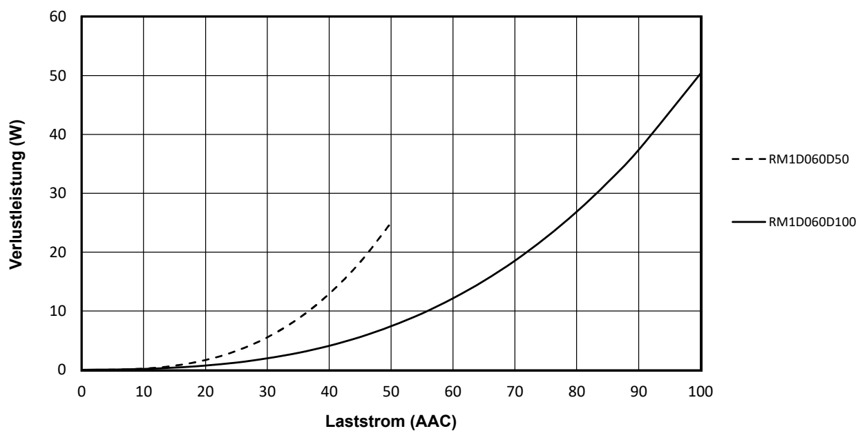
Fig. 8 Verlustleistungskurve
