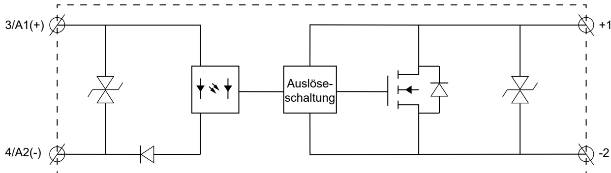
Fig. 10 RM1D Funktionsdiagramm
