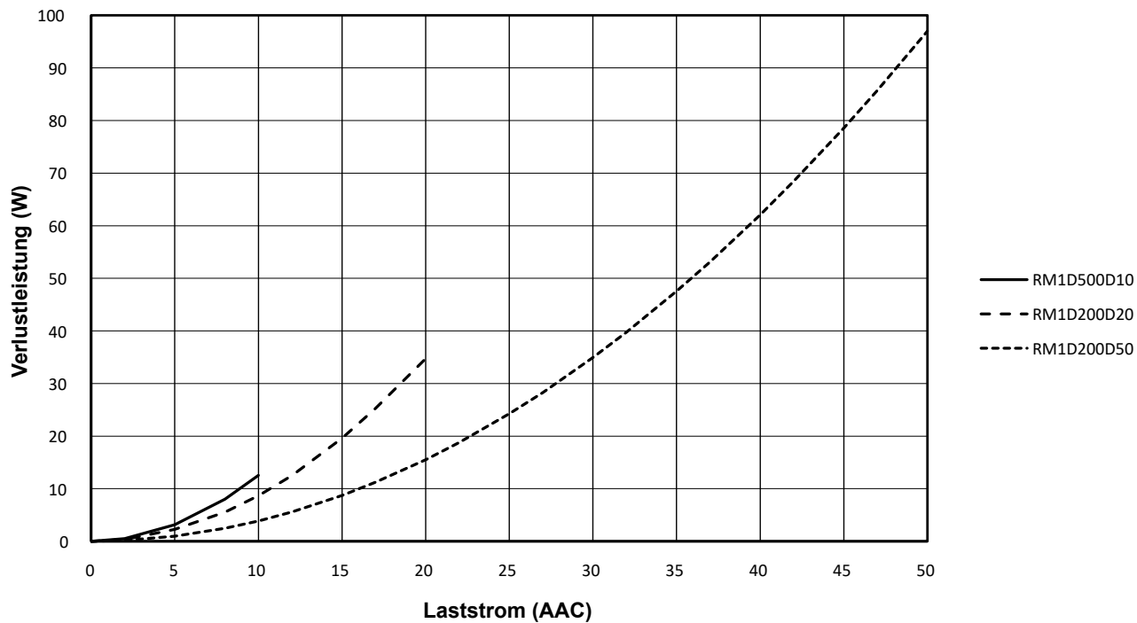
Fig. 9 Verlustleistungskurve
