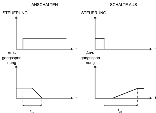
Fig. 2 Reaktionszeitmerkmale
