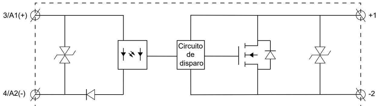
Fig. 11 Diagrama de funcionamiento de la serie RM1D
