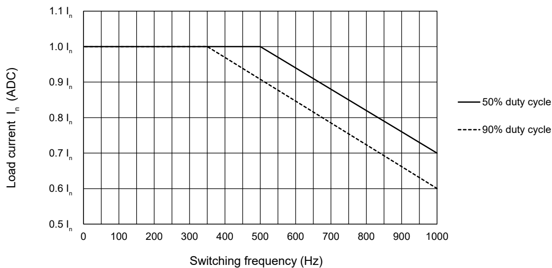
Fig. 4 Curva de intensidad vs. frecuencia de conmutación
