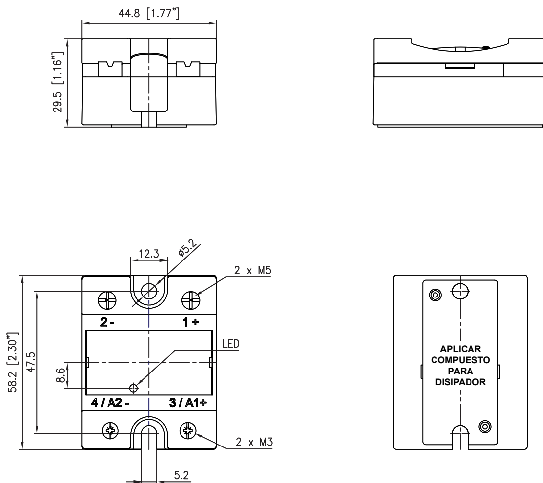
Fig. 1 Dimensiones RM1D
