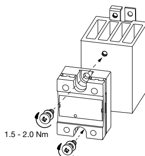
Fig. 13 Avvitare, alternativamente, le viti con una coppia di 0.5 Nm e quindi proseguire con coppia massima di 2.0 Nm.
