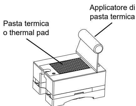
Fig. 12 Uno strato sottile di pasta siliconica termicamente conduttiva deve essere uniformemente distribuito alla base dell'SSR prima del montaggio su un dissipatore di calore. In alternativa, è possibile utilizzare un pad termico. Il materiale dell'interfaccia termica influisce sulle prestazioni termiche. Assicurarsi che il dissipatore di calore sia dimensionato correttamente.
