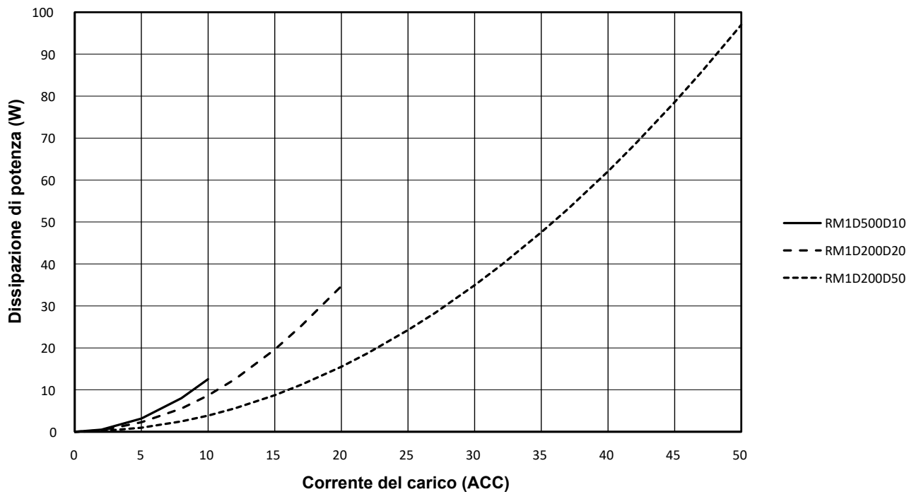
Fig. 9 Grafico di dissipazione della potenza di uscita
