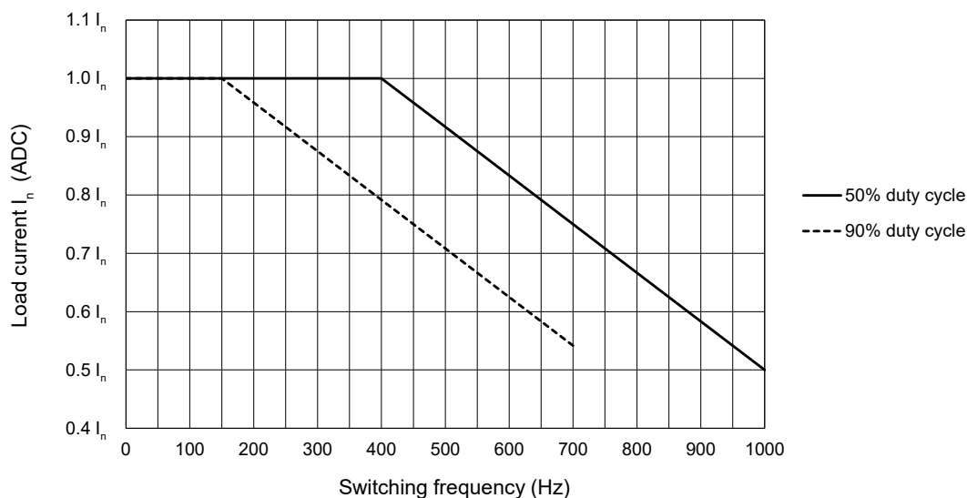
Fig. 5 Corrente di declassamento vs. frequenza di commutazione 4
