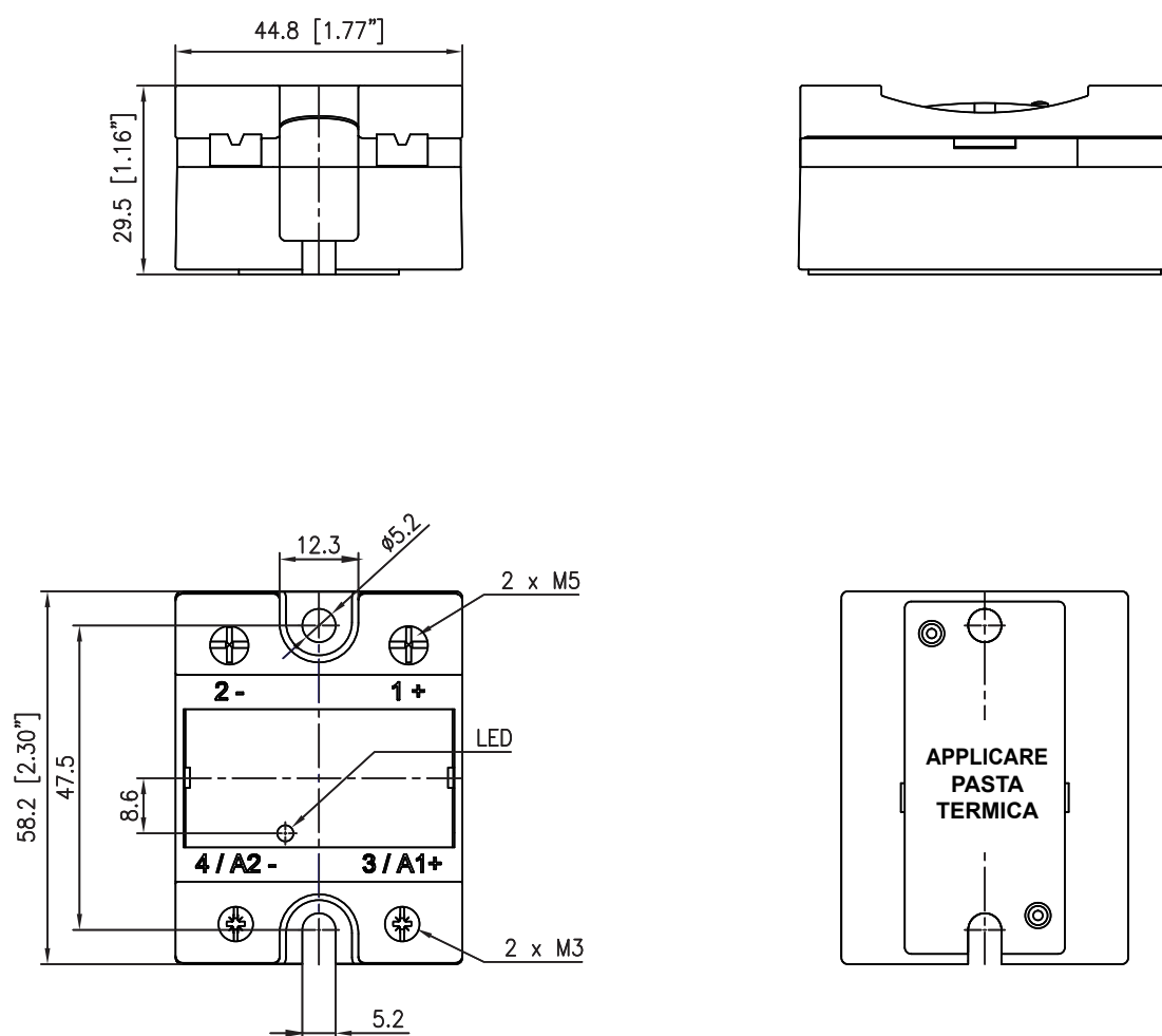
Fig. 1 Dimensioni RM1D
