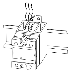
Fig. 14 Montare con le alettature in posizione verticale in modo da garantire un flusso di aria ottimale attraverso il dissipatore di calore.
