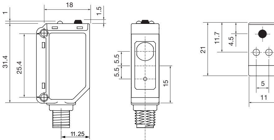
图表 9 插头
