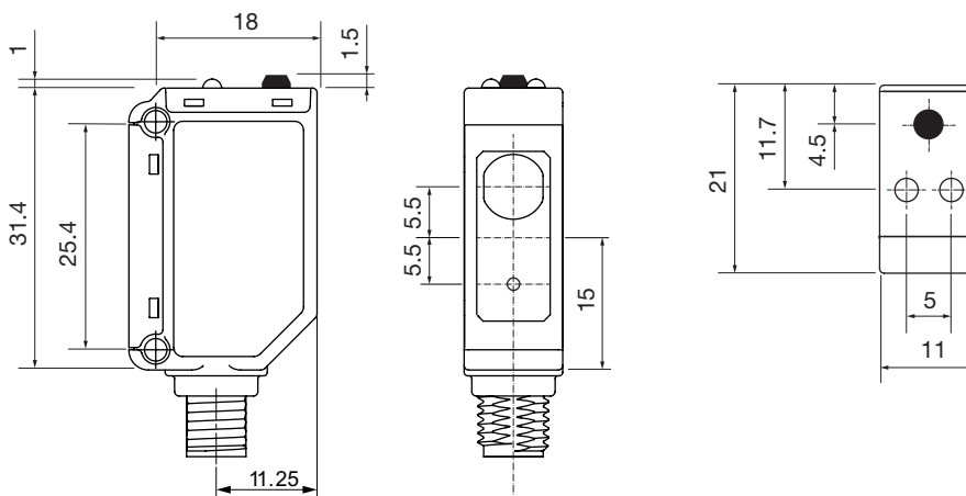
图表 9 插头
