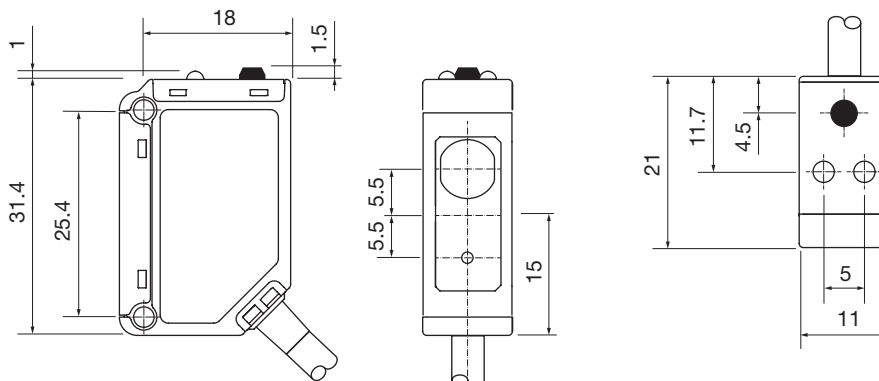
图表 8 线缆
