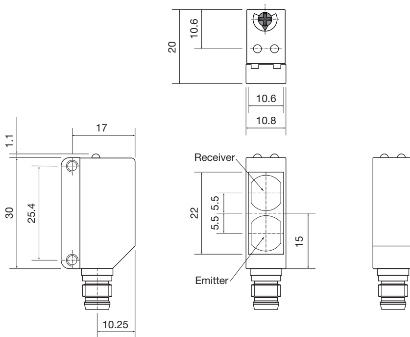
图表 6 插头
