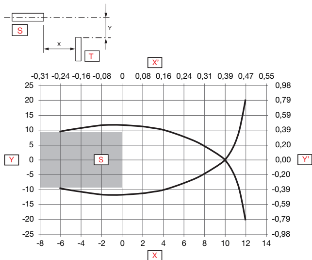
Fig. 5 No empotrado
