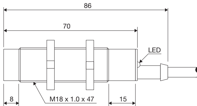
Fig. 7 Cable CA18CAN...A2IO
