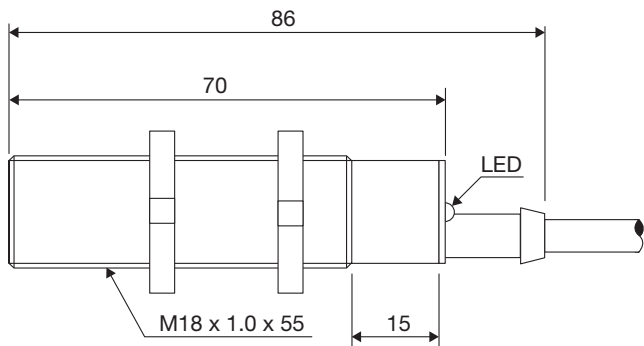
Fig. 6 Cable CA18CAF...A2IO
