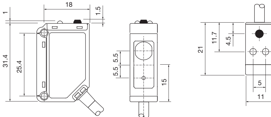
Fig. 9 Cable
