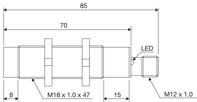
Fig. 9 Conducteur CA18CAN...M1IO
