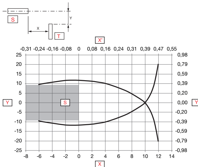
Fig. 5 Non affleurant
