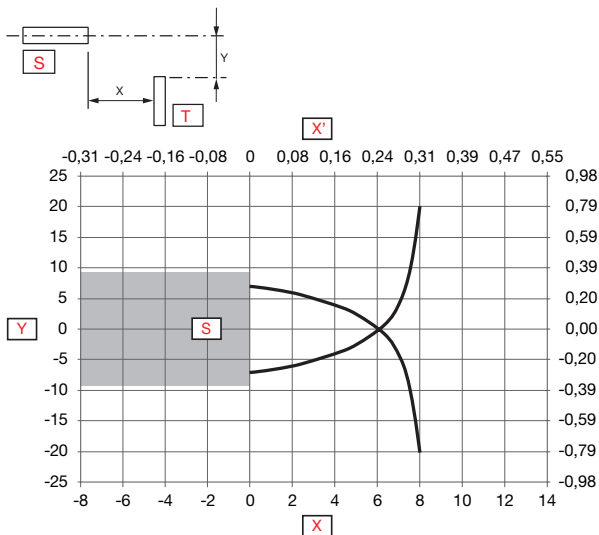
Fig. 4 Affleurant
