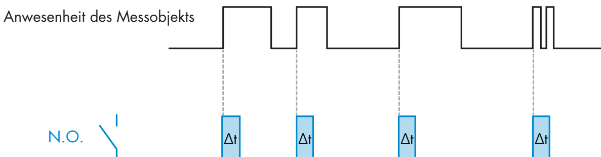
Beispiel mit Schließerausgang
