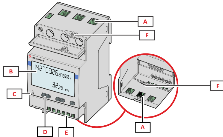
Abb. 1 Vorderseite
