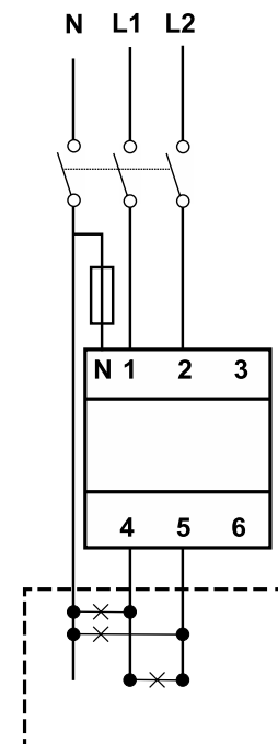
Abb. 5 Zweiphasen-System mit Nullleiter (3 Adern)
