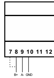
Abb. 10 Letztes Gerät auf RS485
