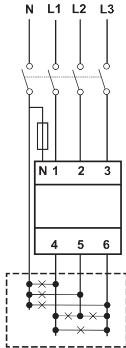
Abb. 3 Dreiphasig mit Nullleiter (4-drahtig)
