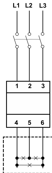
Abb. 4 Dreiphasig ohne Nullleiter (3-drahtig) MID
