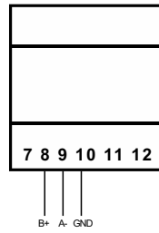
Abb. 9 RS485-Anschluss
