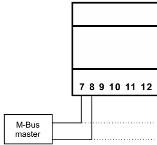
Abb. 8 M-Bus
